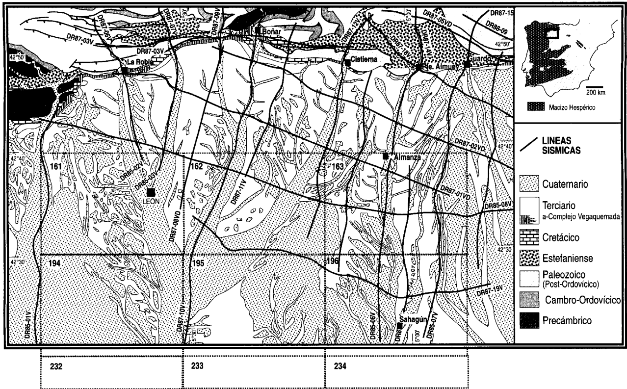
Fig. 9.- Situación de las líneas sísmicas realizadas por REPSOL en el borde noroccidental de la Cuenca del Duero.
