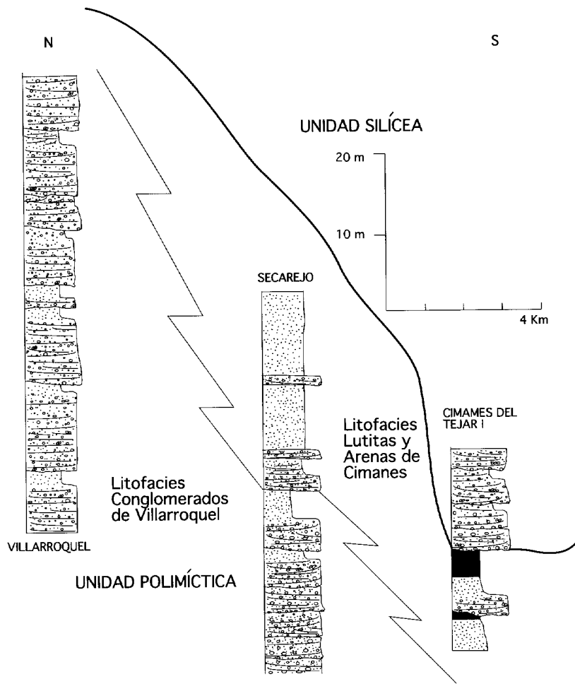
Fig. 5.- Correlación entre diversas secciones estratigráficas de la Hoja de León.
