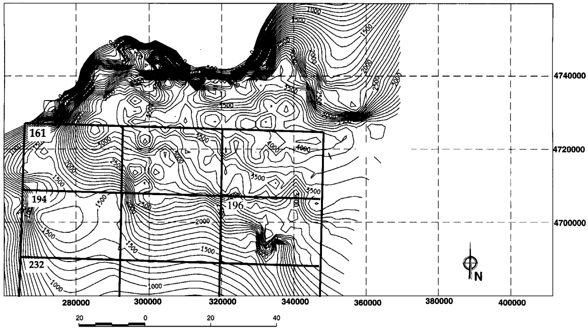
Fig. 13.- Mapa de Isobatas del Techo de Basamento-Base del Mesozoico. Intervalo de contomos: 100m. Según Redondo et. al. (1995).
