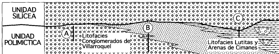
Columnas estratigráficas A-Villarroquel, B-Secarejo y C-Cimanes del Tejar I.
