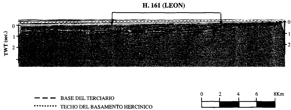
Fig. 10.- Interpretación geológica del perfil sísmico DR85-01V. Situación en la Fig.9. Según Redondo et. al. (1995), ligeramente modificada.
