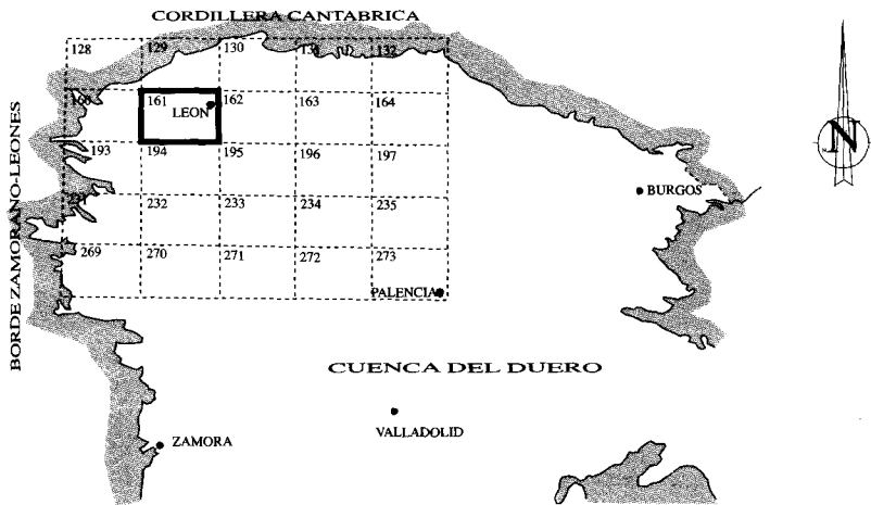
Fig. 1.- Situación de la Hoja Nº 161 (León) en el ámbito de la Cuenca del Duero.
