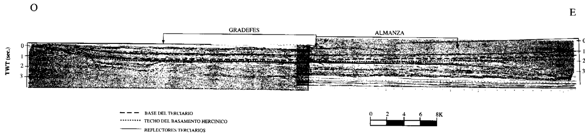
Fig. 11.- Interpretación geológica del perfil sísmico DR85-08V. Situación en la Fig.9. Según Redondo et. al. (1995), ligeramente modificada.
